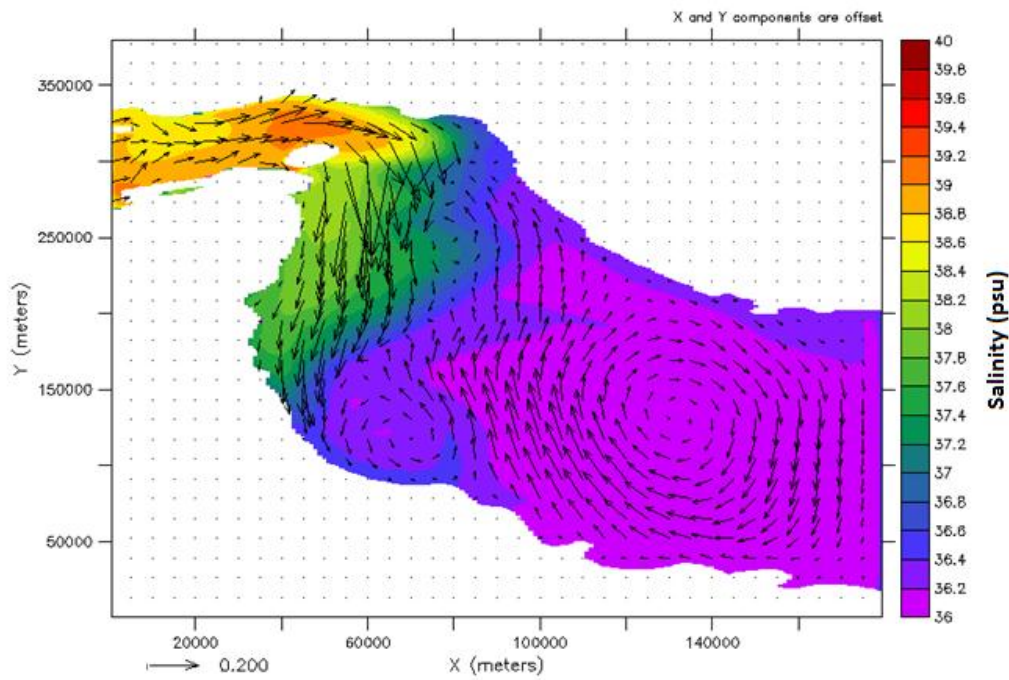
شکل ۷. بردارها گردش آب دریای عمان را در عمق ۵۰ متری نشان می دهند. رنگ زمینه نیز شوری آب در این عمق را نشان می دهد. این شکل، خروج آب شور خلیج فارس به دریای عمان را از طریق تنگه هرمز در لایه زیر سطح تأیید می کند. همچنین این شکل نشان می دهد که گردش آب در این عمق نیز شبیه آب های سطحی است.
